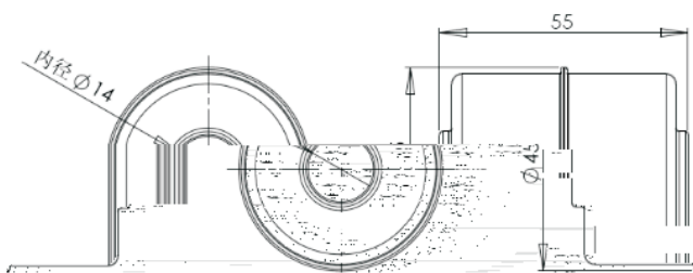
带显示磁性浮球外形尺寸图
